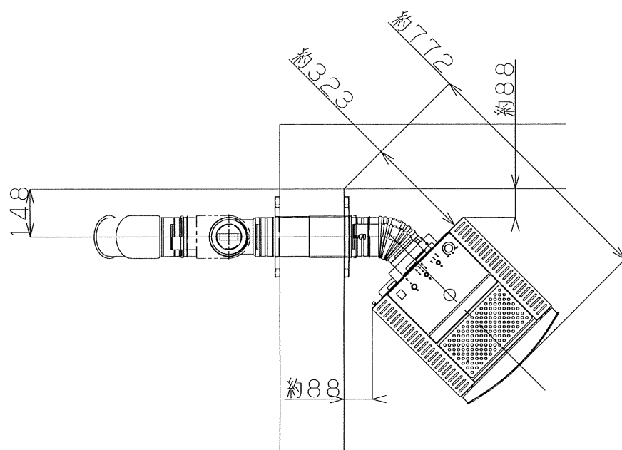
PE-6 設置図
