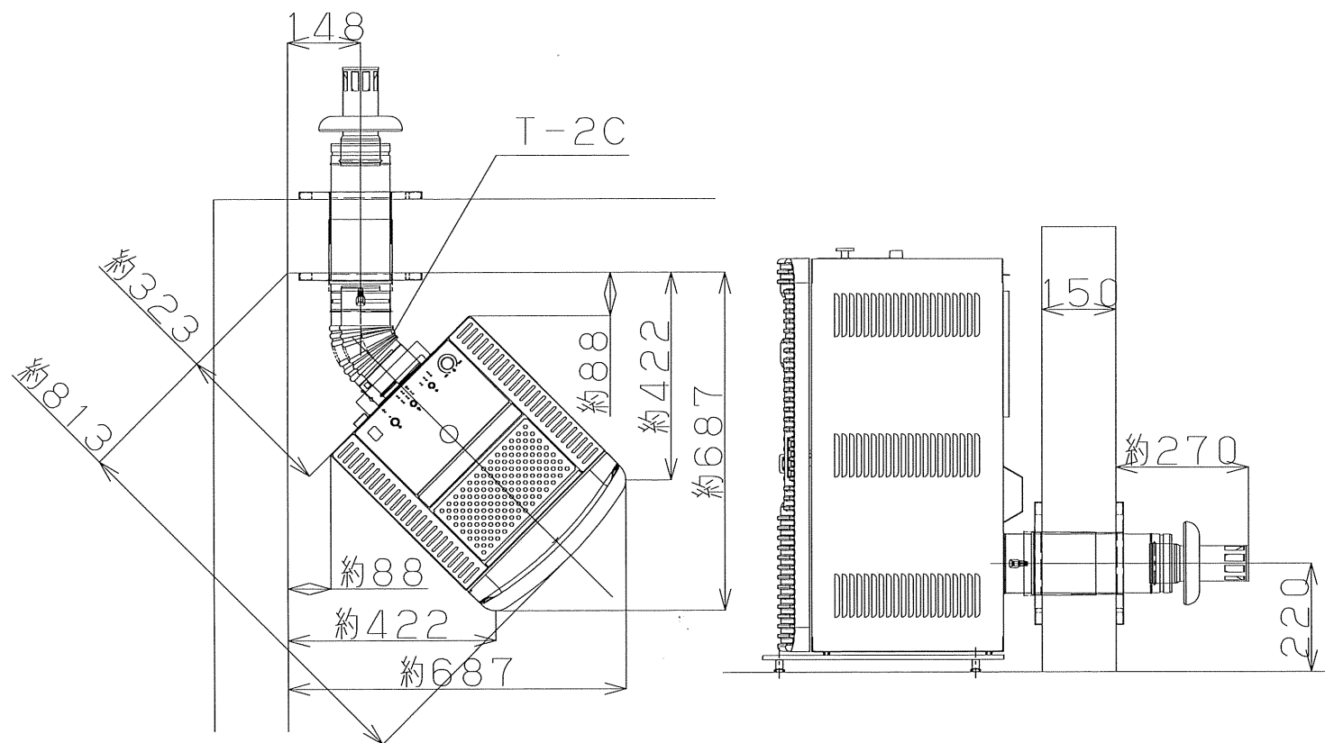
PE-6CT標準設置図
