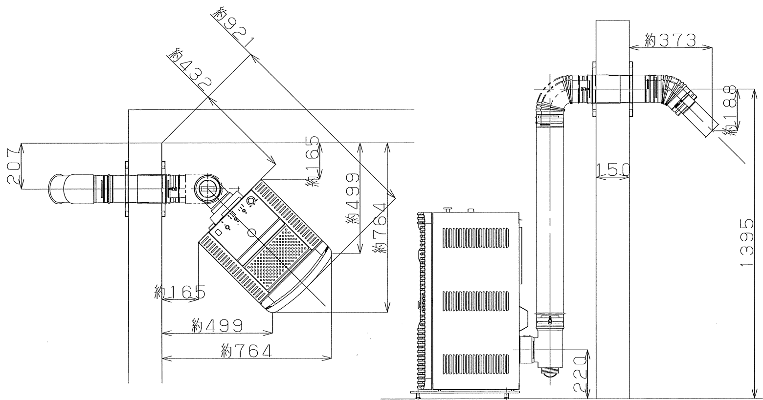
PE-6CT標準設置図
