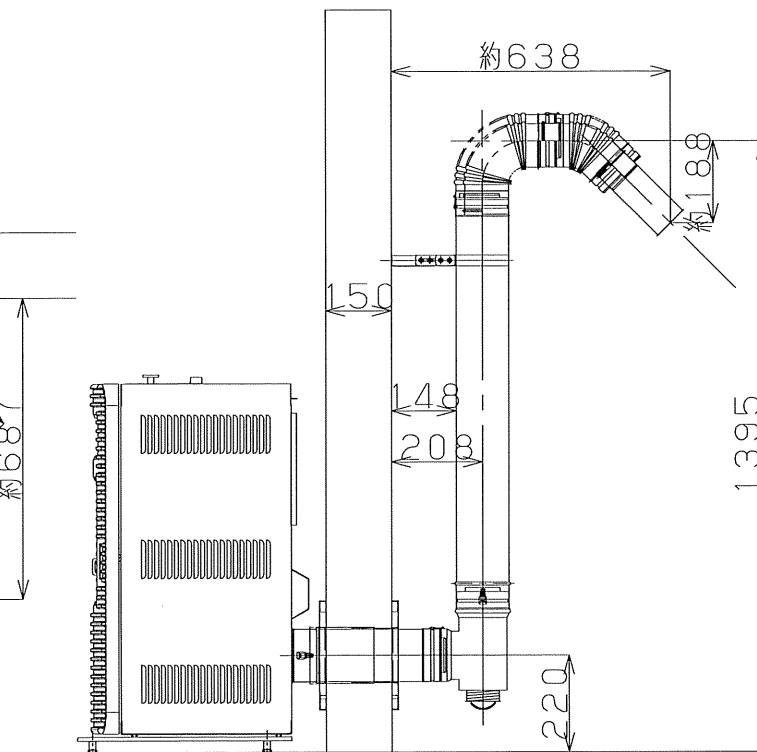
PE-6CT 標準設置図
