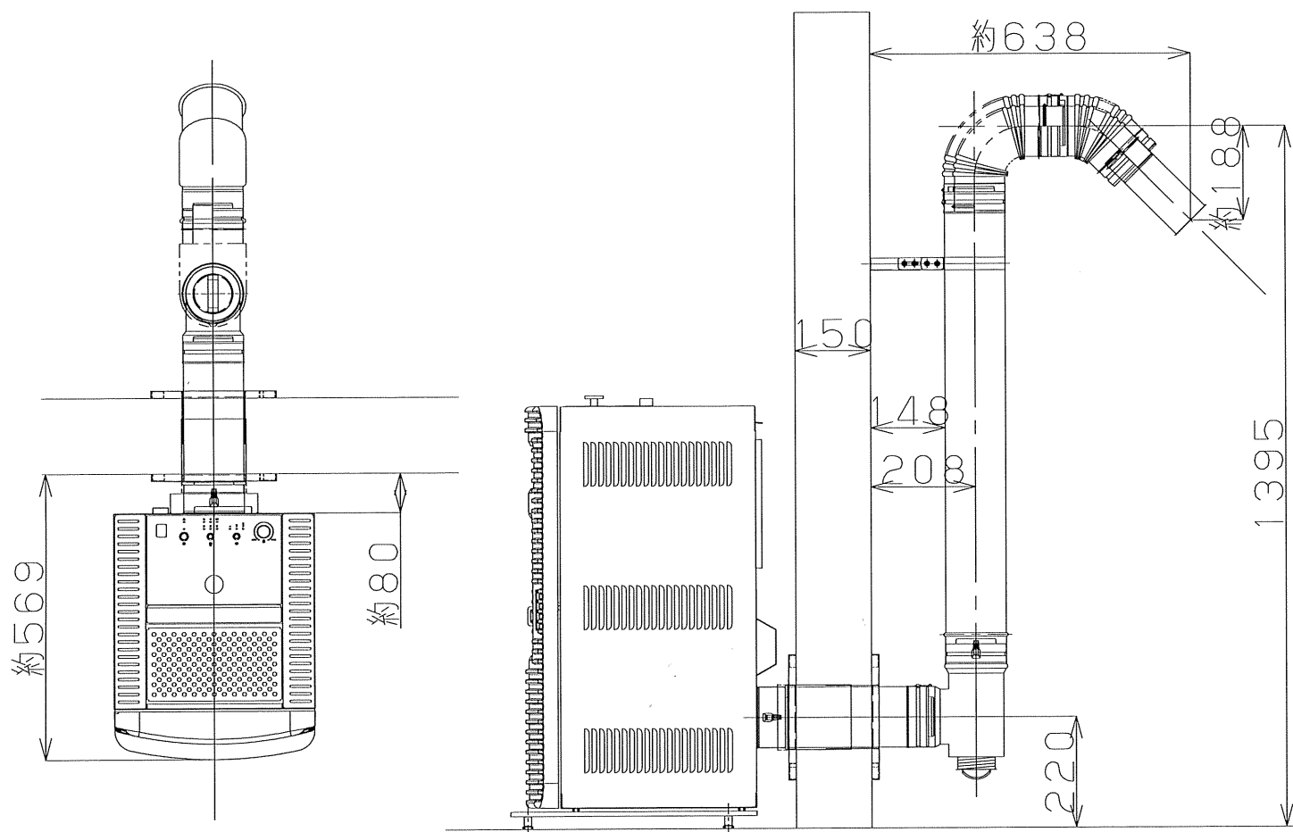
PE-6CT標準設置図
