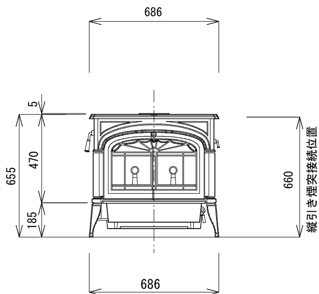
立面図
