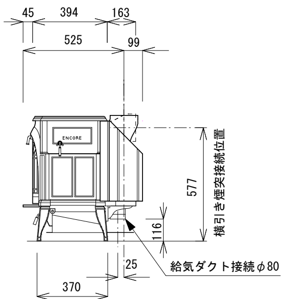
側面図
