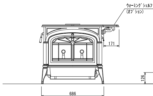
正面図
