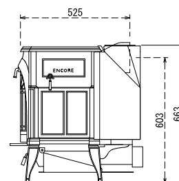
側面図(8インチ)
