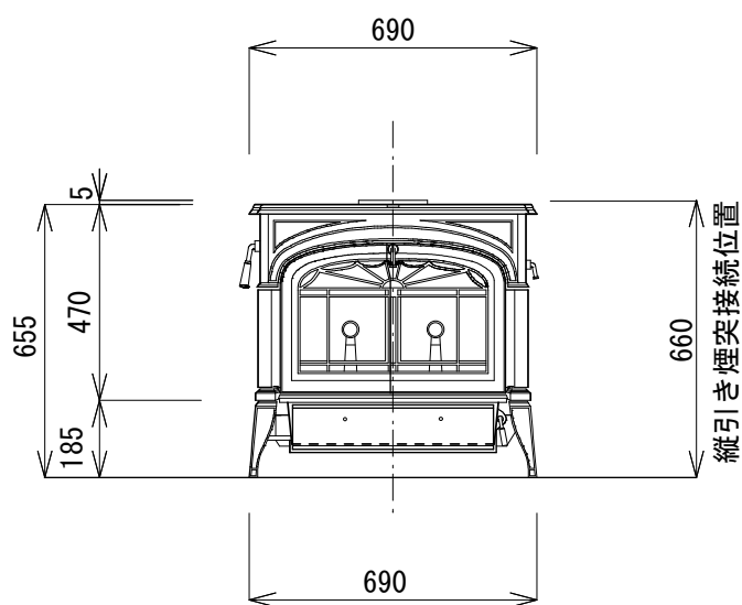
立面図
