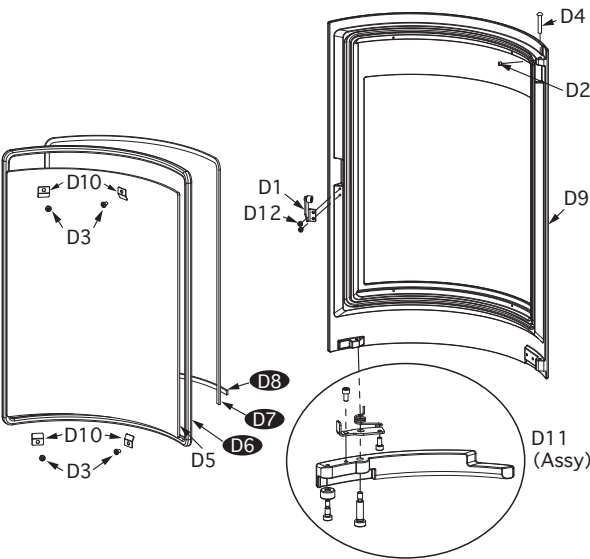
灰受けドア
