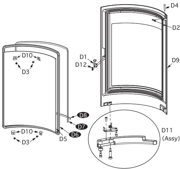
灰受けドア
