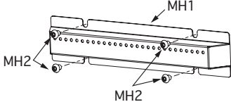
MH 拡大図
