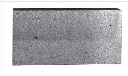
品名：ピキャン用標準ブリック 品番：Y5106500 寸法：115×230×t=40 mm 単位：1枚（1台あたり9枚必要）
