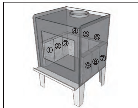
品名：ピキャン用標準ブリック 品番：Y5106500 寸法：115×230×t=40 mm 単位：1枚（1台あたり9枚必要）
