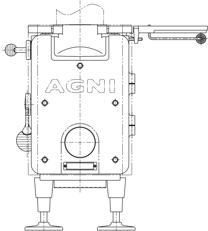
背面図
