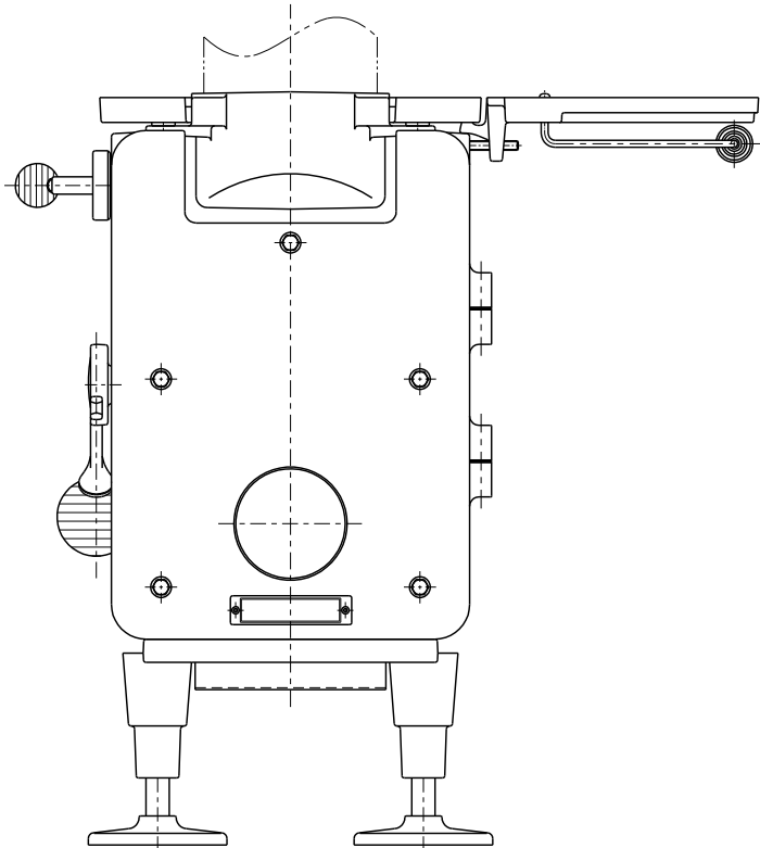
背面図
