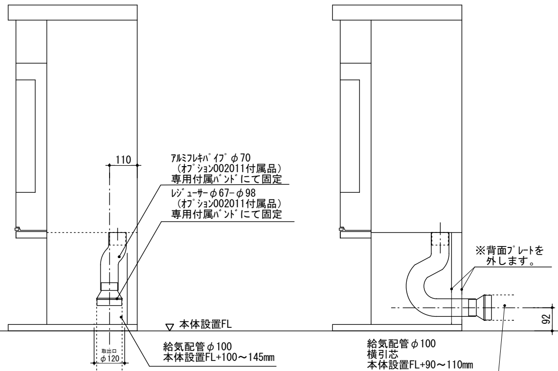
外気取入要領図
