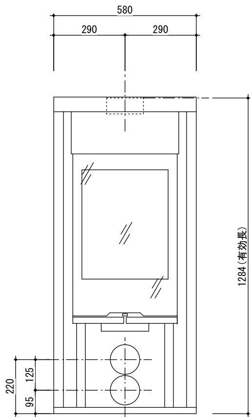
正面図
