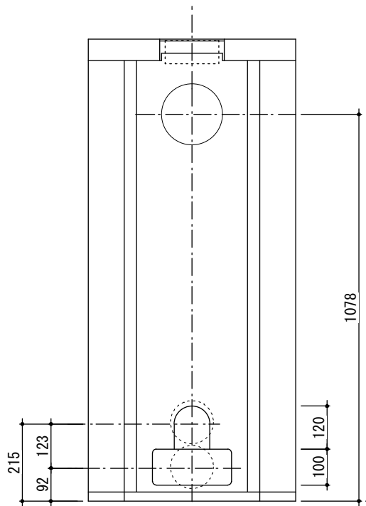
背面図
