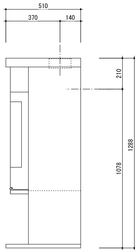
右側面図
