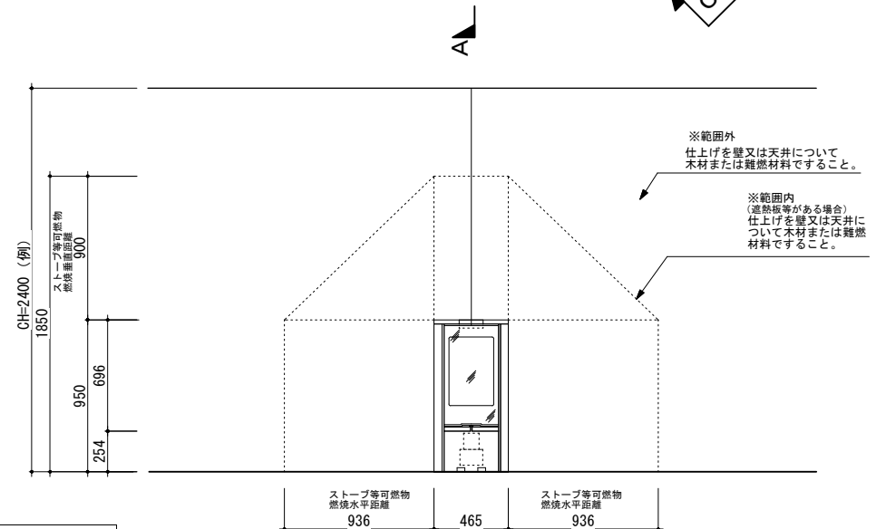
B-B' 断面図
