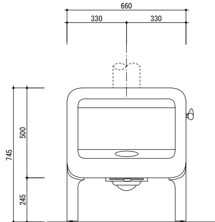
正面図
