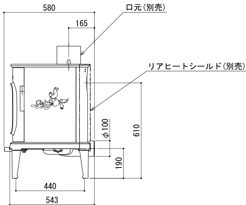
側面図
