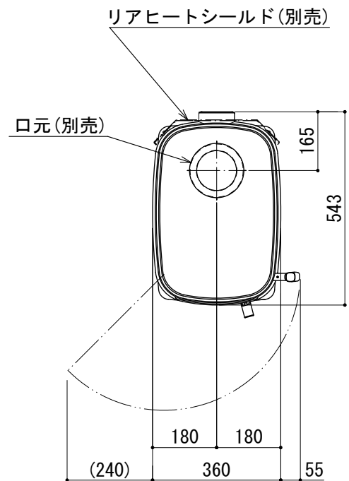
平面図
