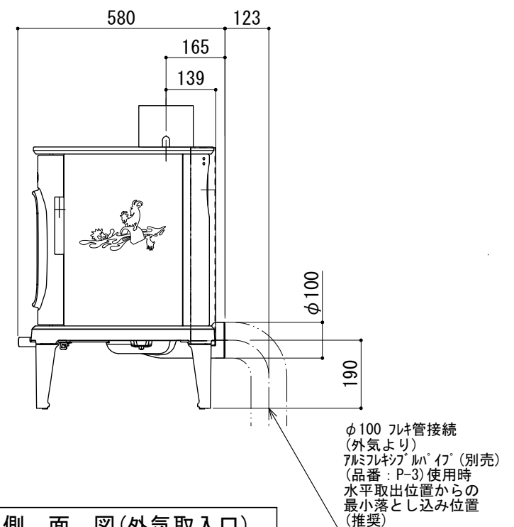
側面図(外気取入口)
