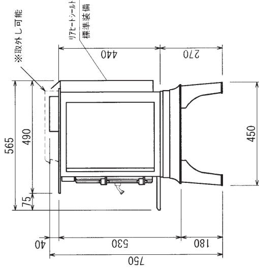
右側面図
