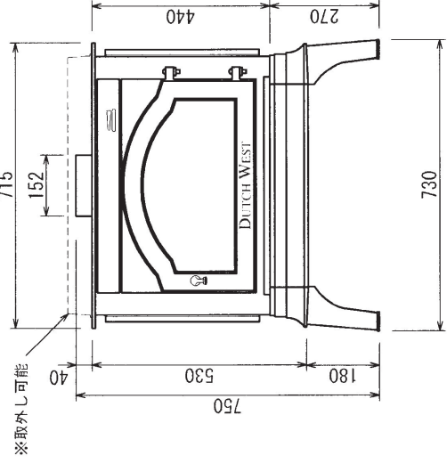
正面図
