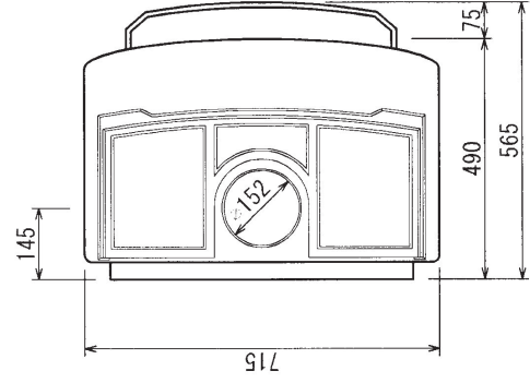
上面図
