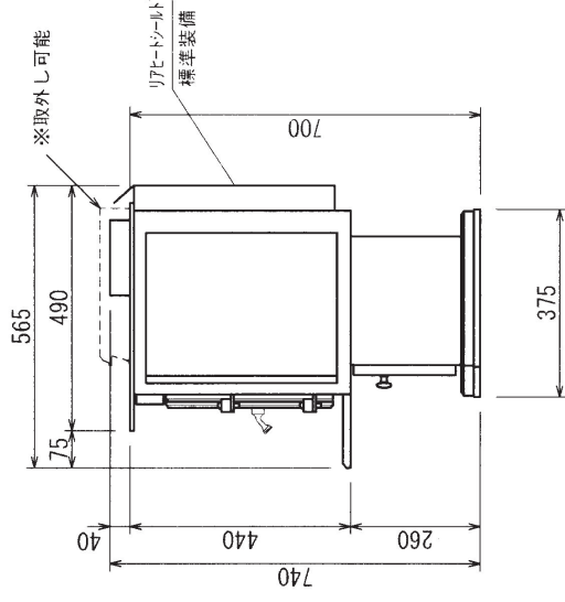
右側面図
