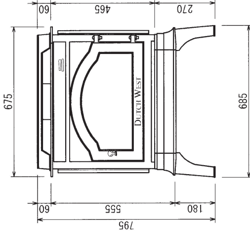
正面図
