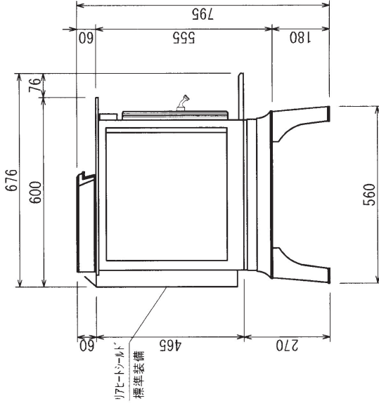
左側面図
