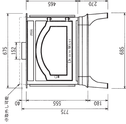
正面図
