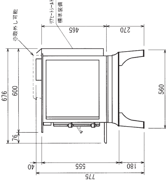
右側面図
