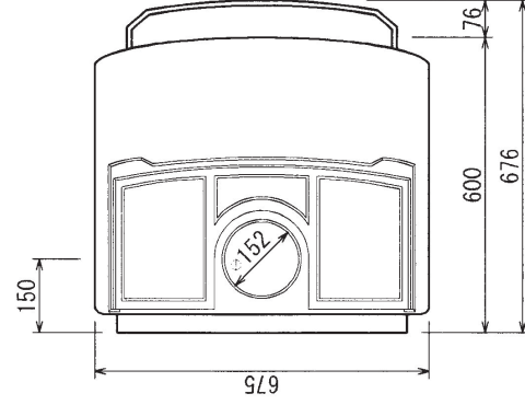
上面図
