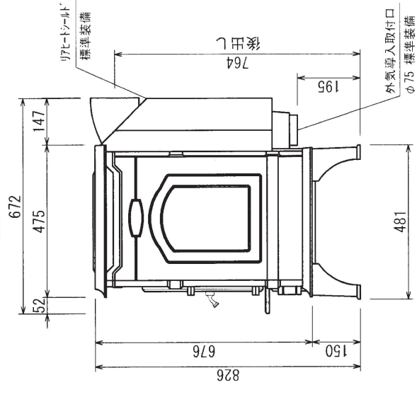
右側面図
