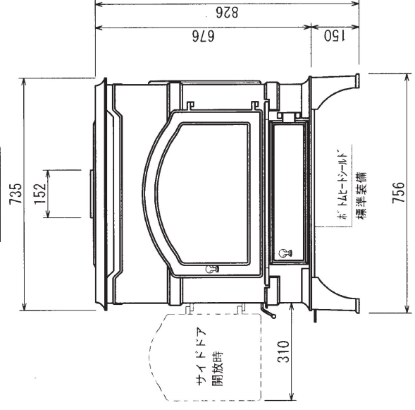
正面図
