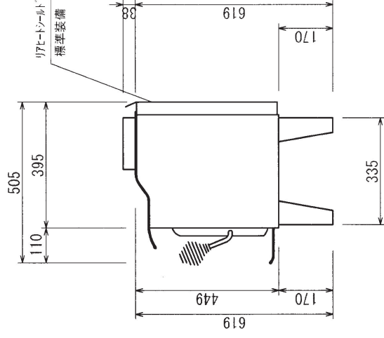
右側面図
