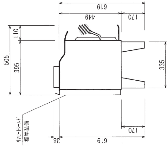
左側面図
