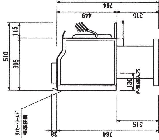
左側面図
