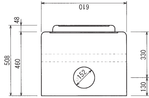
上面図
