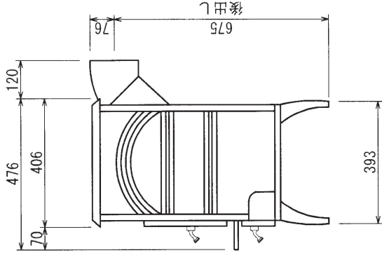
右側面図
