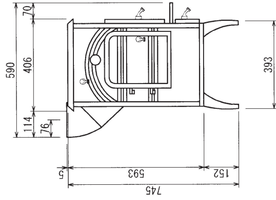
左側面図
