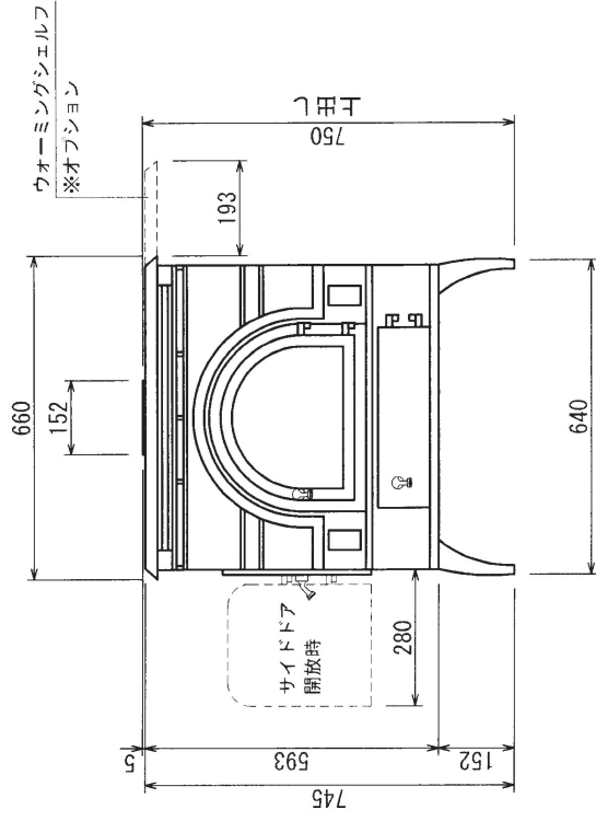
正面図
