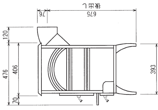
右側面図
