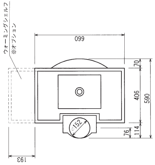
上面図
