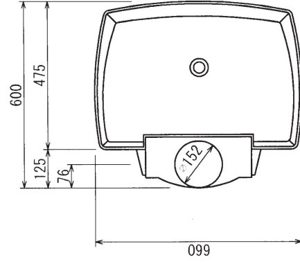
上面図
