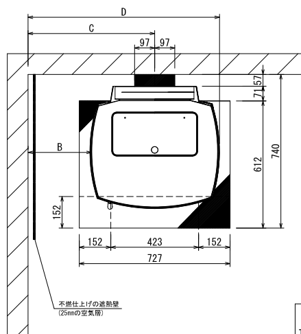
正面図
