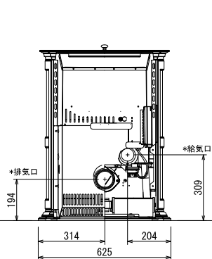
背面図
