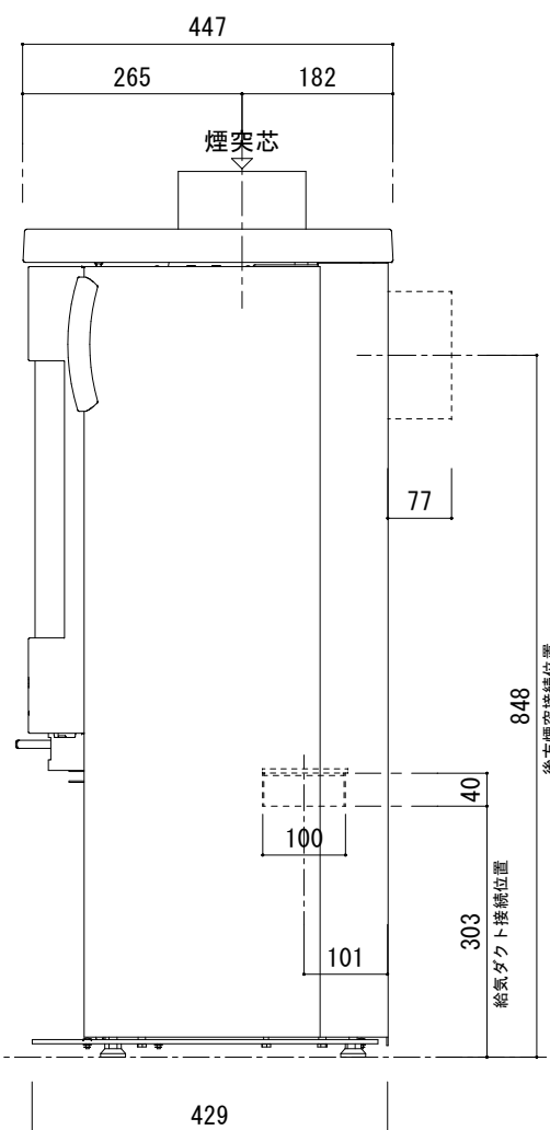
[側面図]
