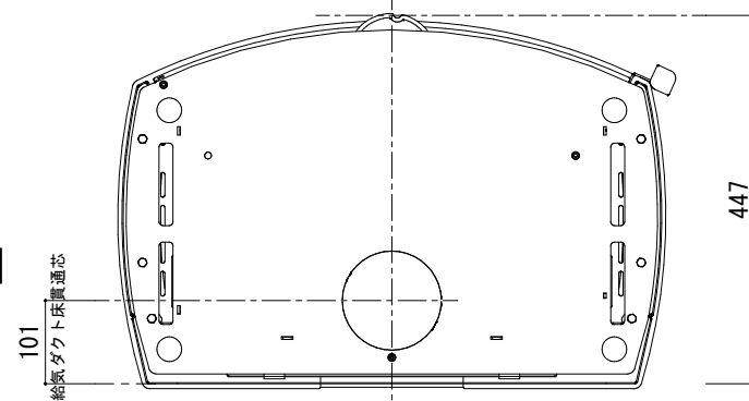
[底面図]
