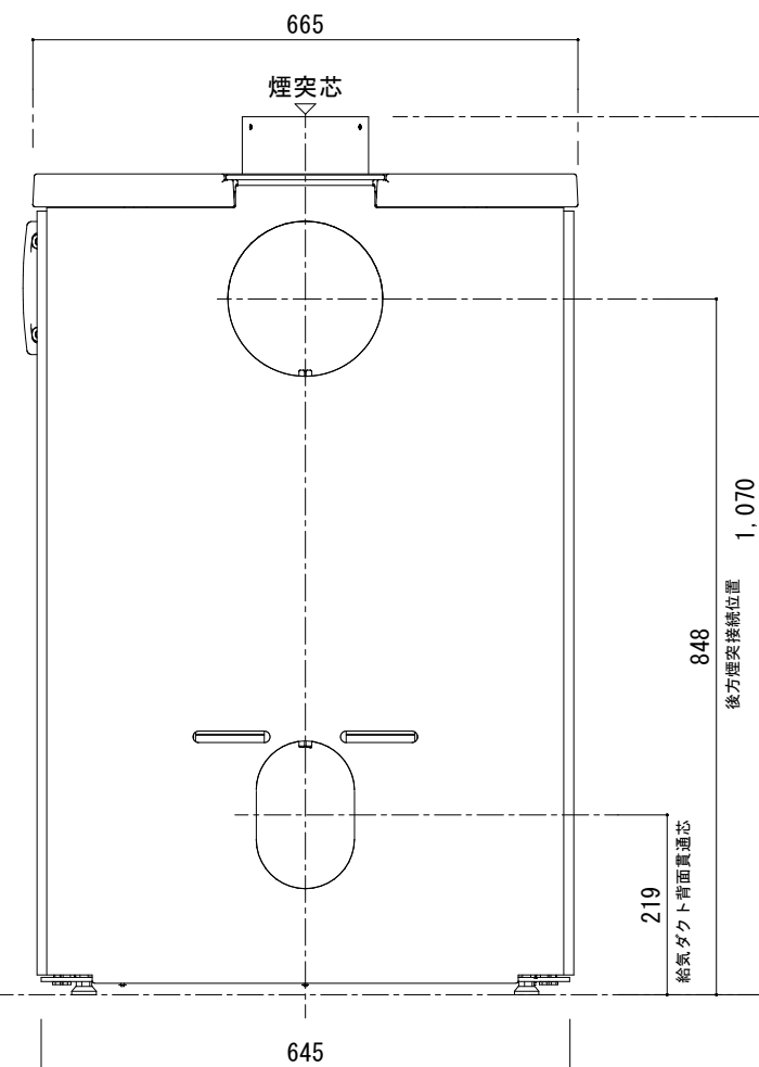
[背面図]
