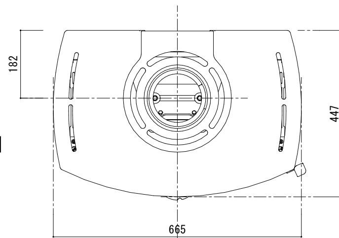
[上面図]
