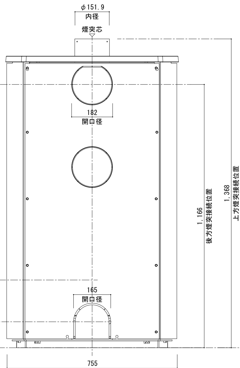
[ 背 面 図 ]
