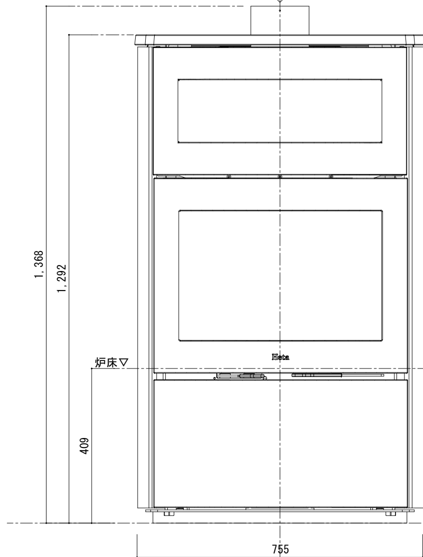
[ 正 面 図 ]
