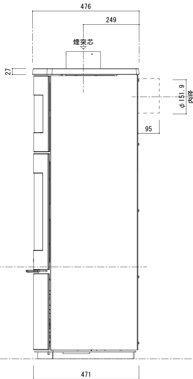
[ 側 面 図 ]
