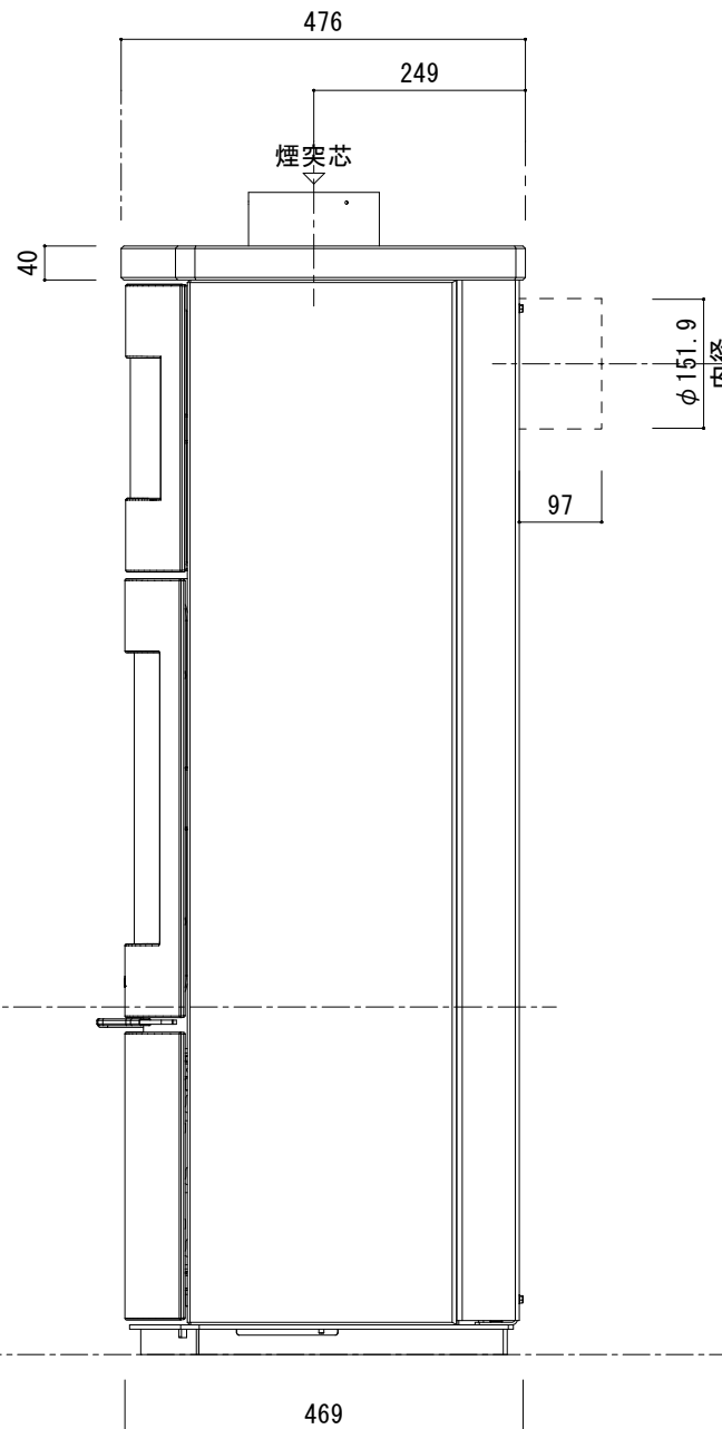
[ 側面図 ]
