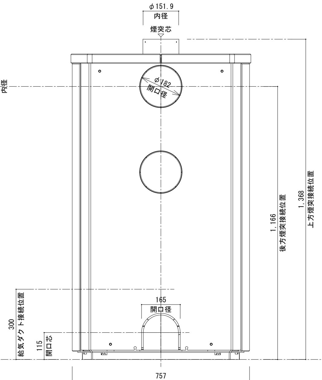
[ 背面図 ]
