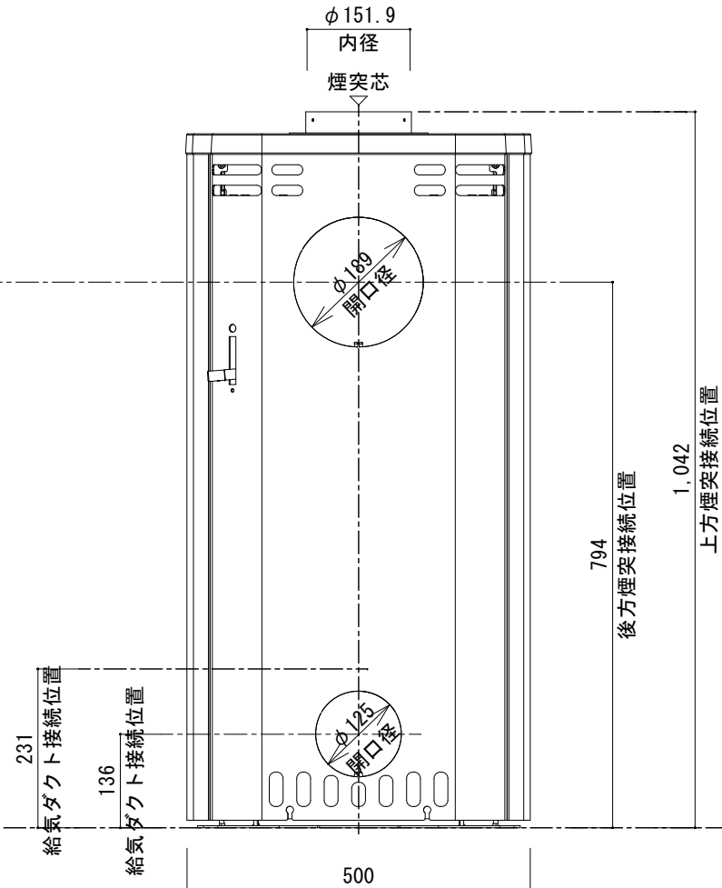
[ 背 面 図 ]
