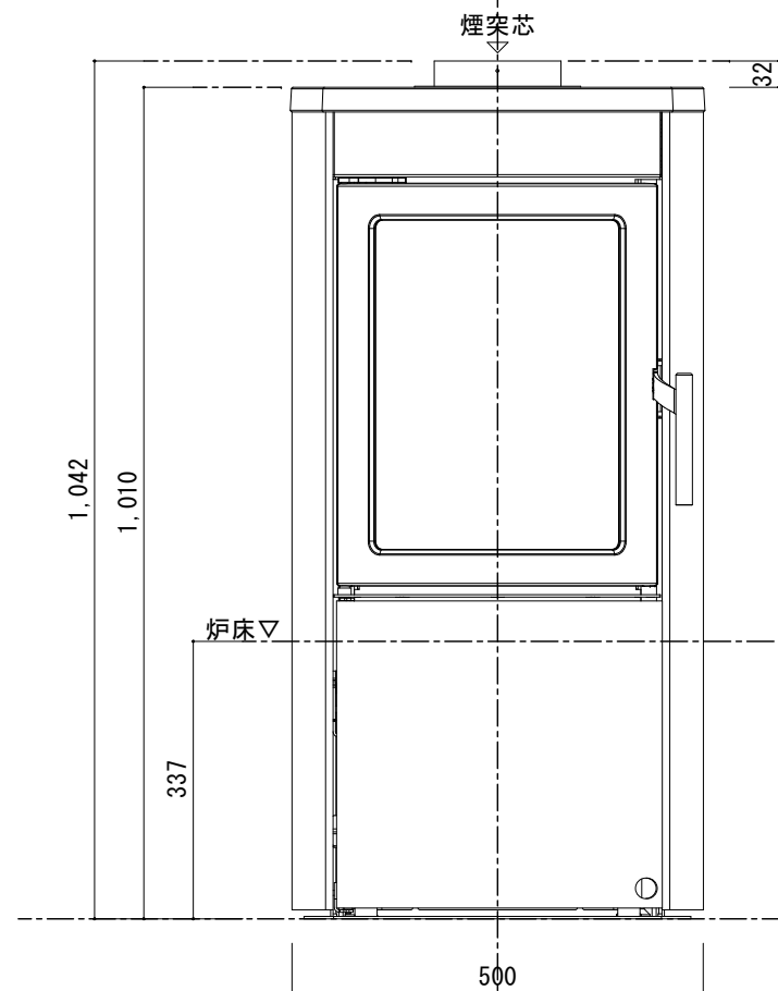
[ 正 面 図 ]
