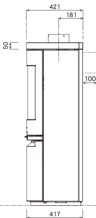
側面図
