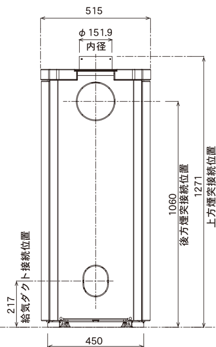
背面図
