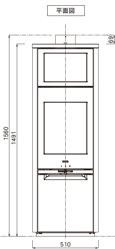
正面図
