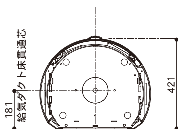
底面図
