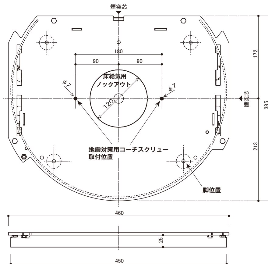
底板正面図
