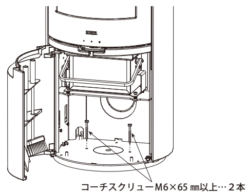
コーチスクリューM6×65 mm以上…2本
