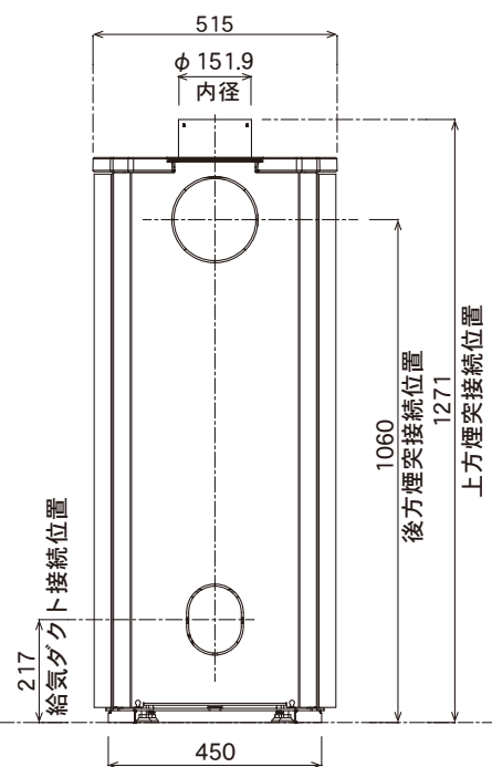
背面図
