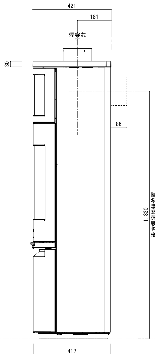
[ 側 面 図 ]
