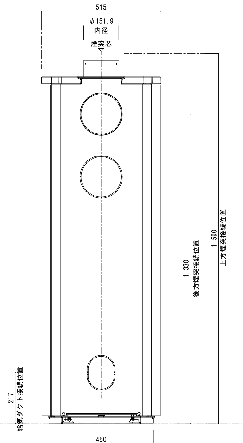
[ 背 面 図 ]
