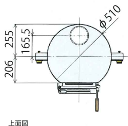
上面図
