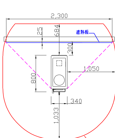
平面図 平行設置
