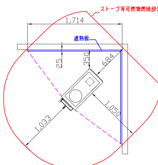
平面図 コーナー設置
