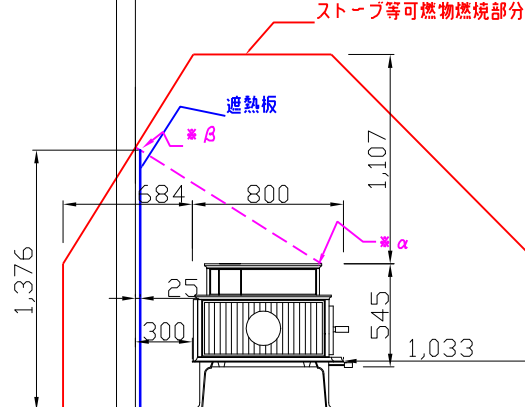
側面図 平行設置
