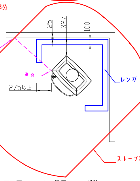
平面図 コーナー設置 レンガ積み
