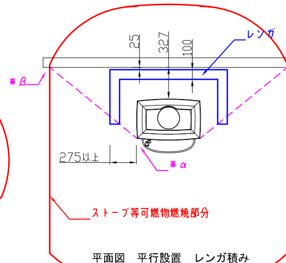
平面図 平行設置 レンガ積み
