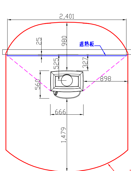
平面図 平行設置
