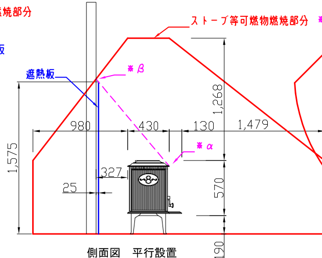
側面図 平行設置
