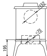
背面図
