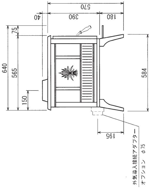
左側面図
