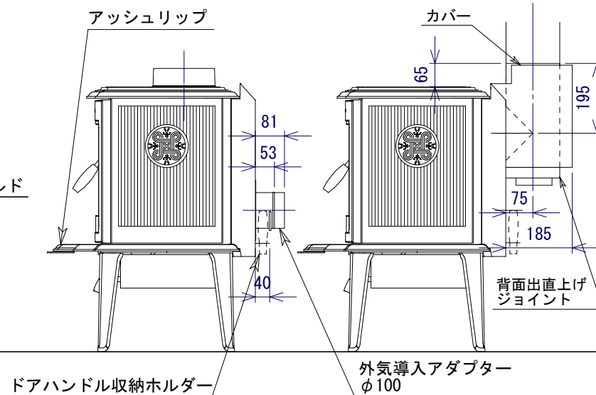
側面図
