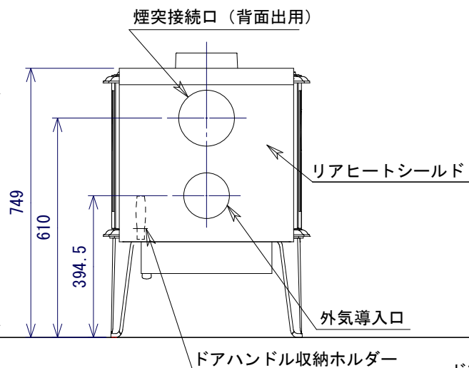
背面図
