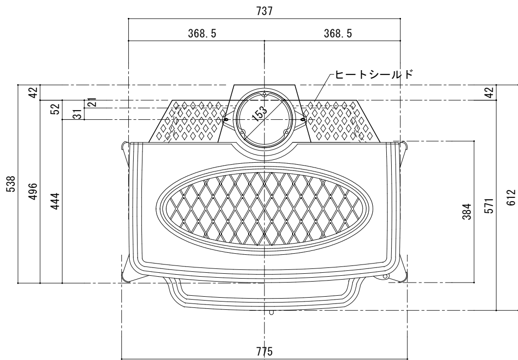
[ 上 面 図 ]
