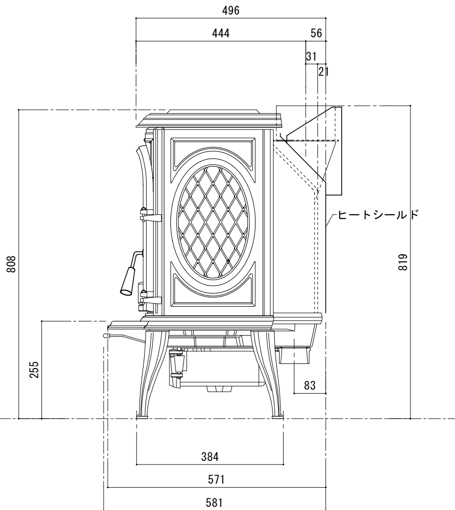
[ 側 面 図 ]
