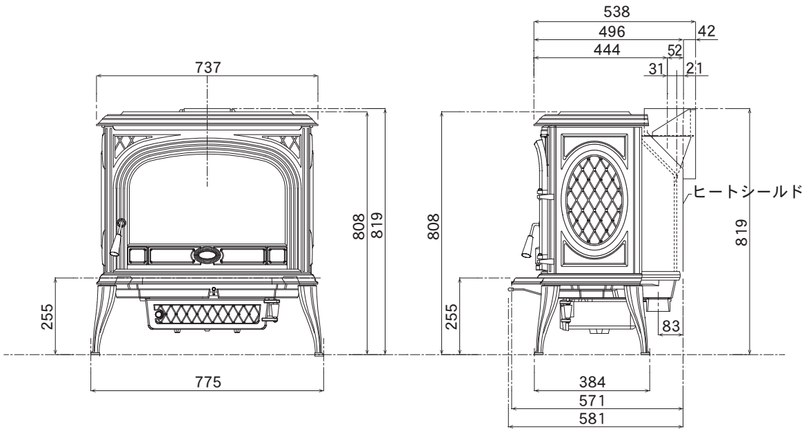
正面図
