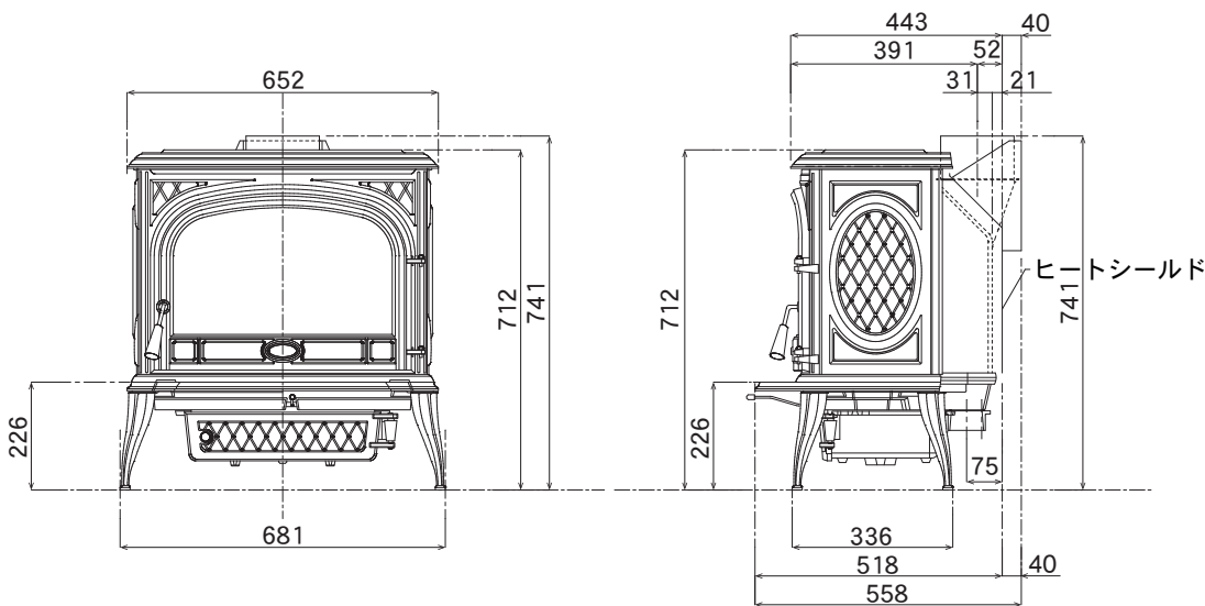
正面図
