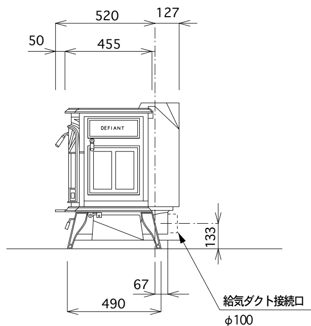
側面図
