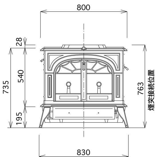
正面図
