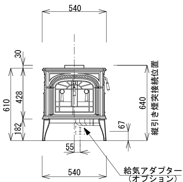
立面図
