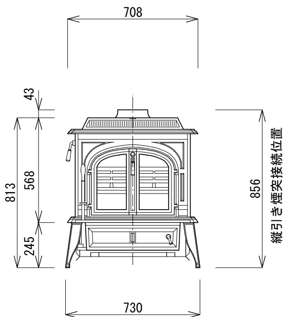
立面図
