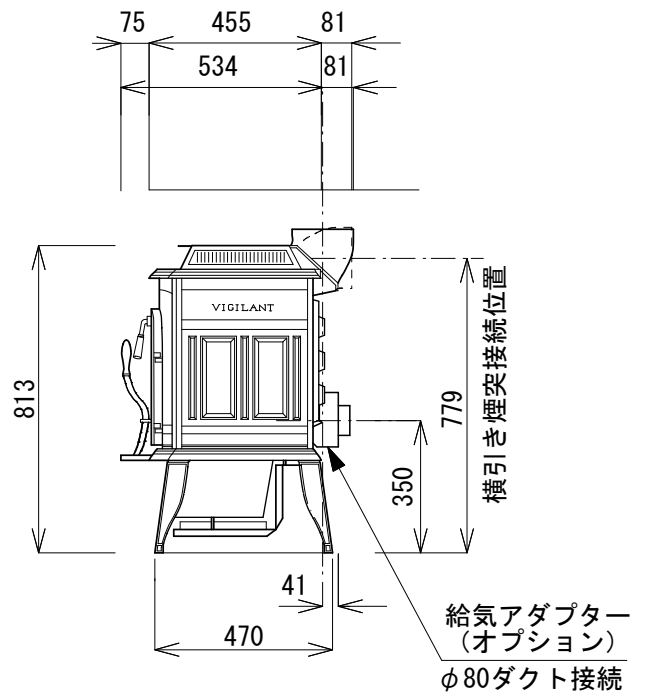
側面図
