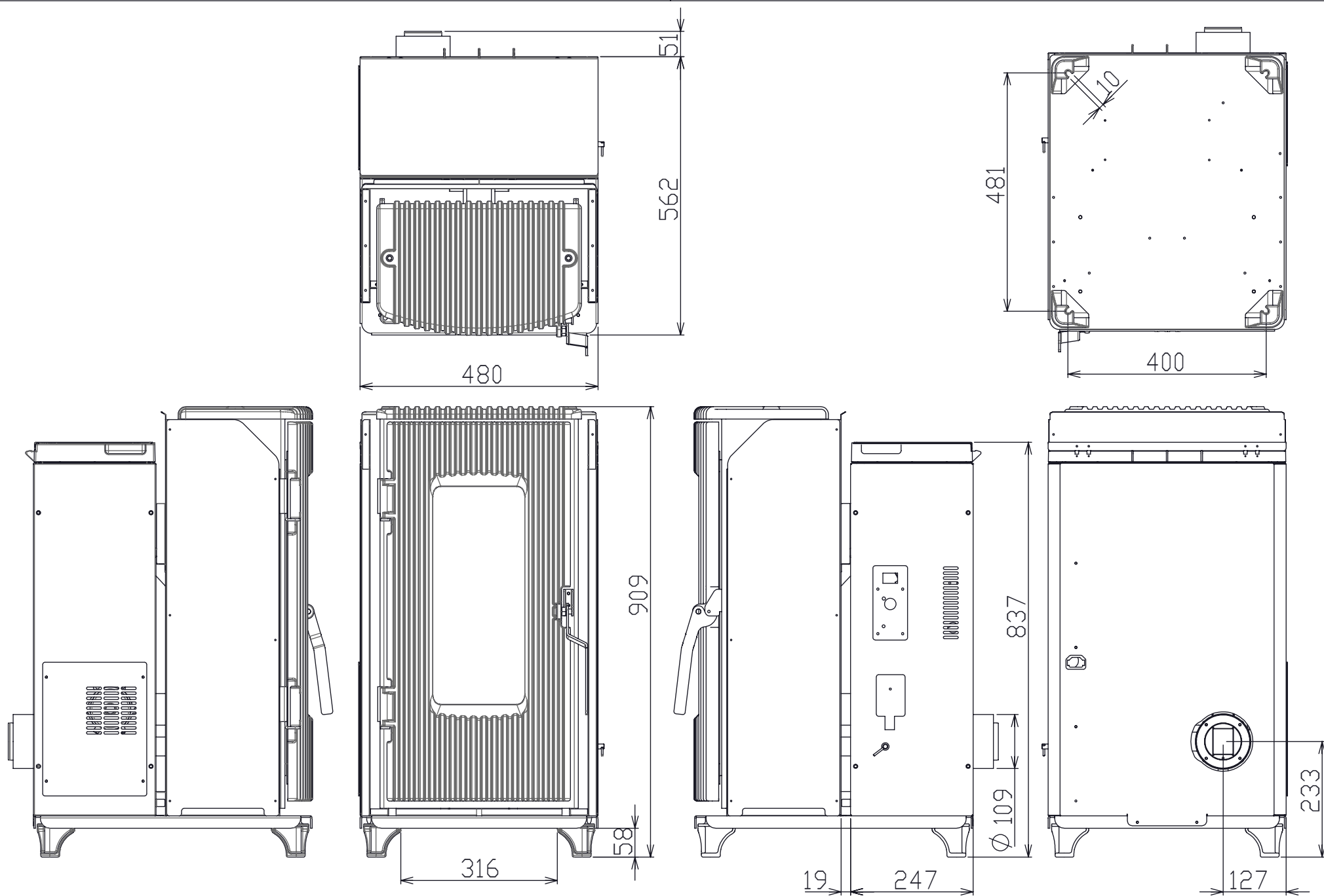
warmArts RS-4 外觀寸法図
