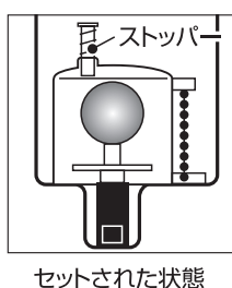
感震自動消火装置図
