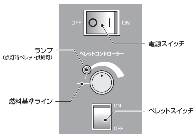
操作盤図
