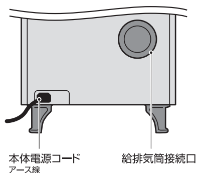
裏面図
