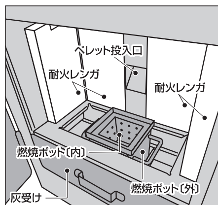
内部図
